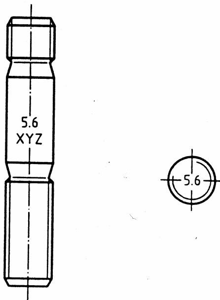
Рисунок 10 – Маркировка шпилек
